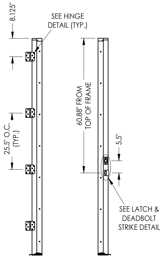
HINGE JAMB
